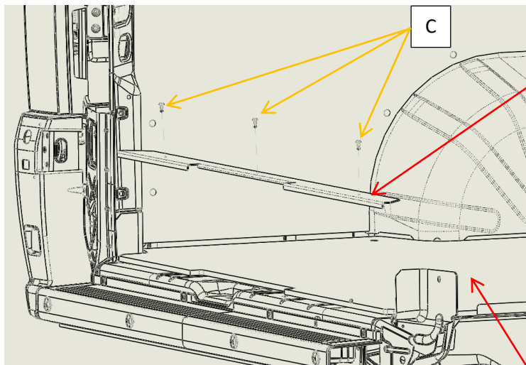
ITEM 18 FLOOR SILL – REAR DOOR
