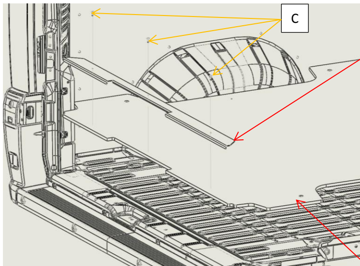
ITEM 18 FLOOR SILL – REAR DOOR
